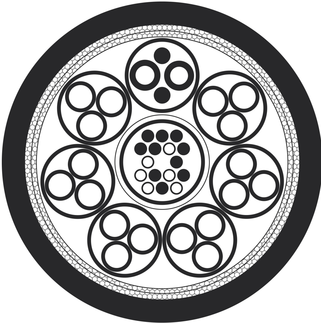
Abb. 2: HRADIL CAN-Bus High Endurance Hybrid Kabel im Querschnitt
