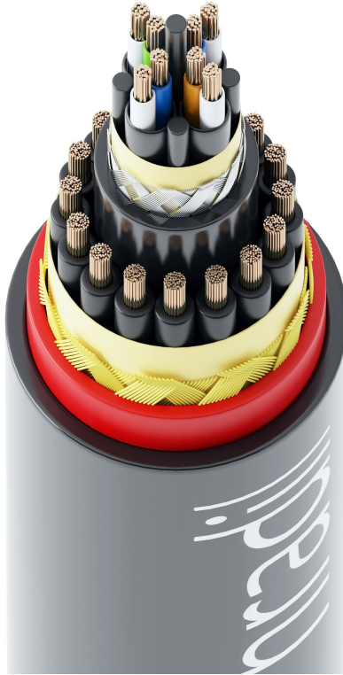
Abb. 3: Das Hradil High-Endurance-Kabel für Eisenbahnfahrzeuge im Querschnitt.
