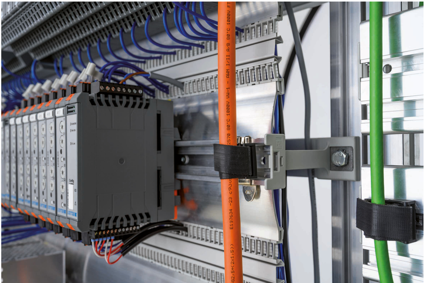
Abb. 1: Klettbandsocket von LÜTZE zur vertikalen Leitungsverlegung über die Tragschiene (VPSym) oder Stegprofile
